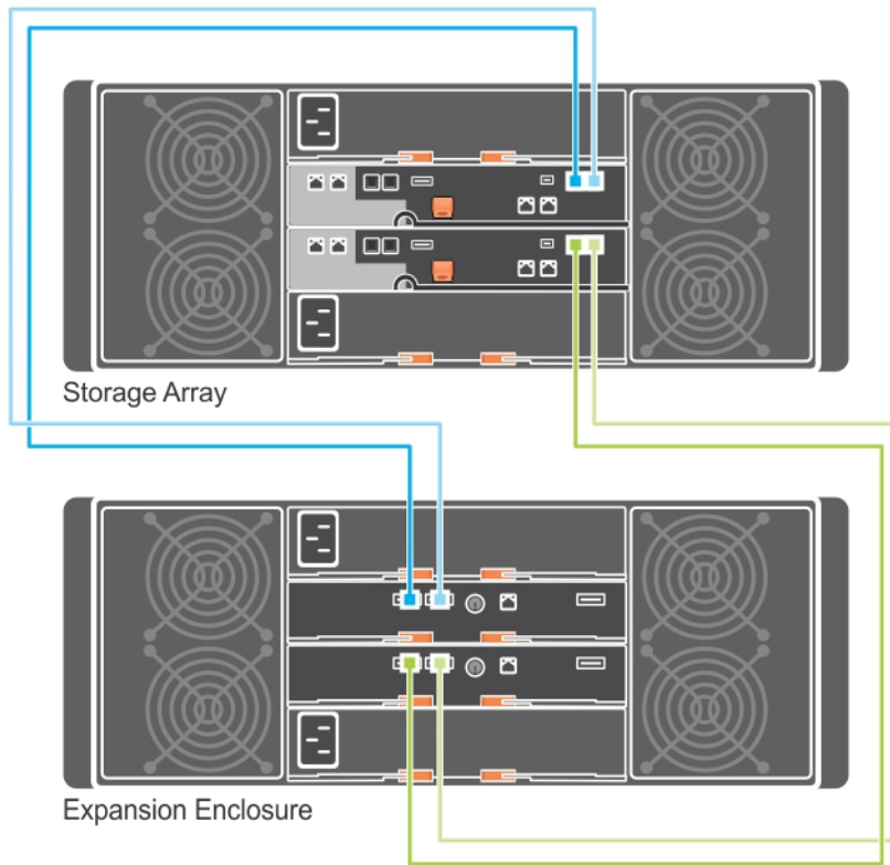
그림 7. 단일 확장 다이어그램
