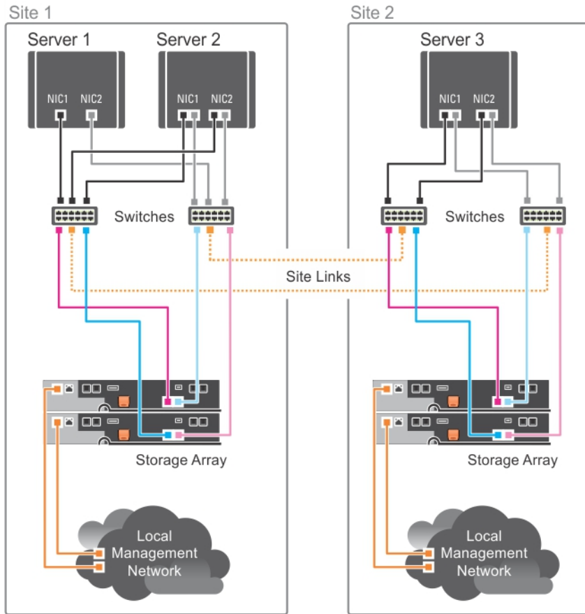
그림 5. 원격 복제 환경
