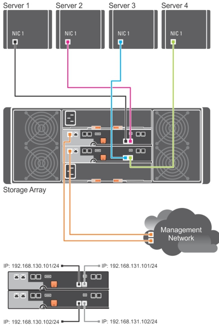
그림 1. 이중 컨트롤러 구성의 호스트 4개
